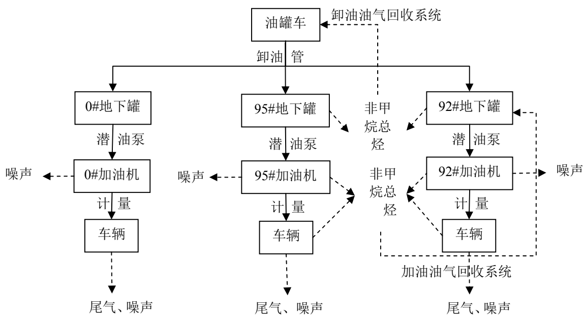
图 3-1 项目工艺流程及产污位置图
