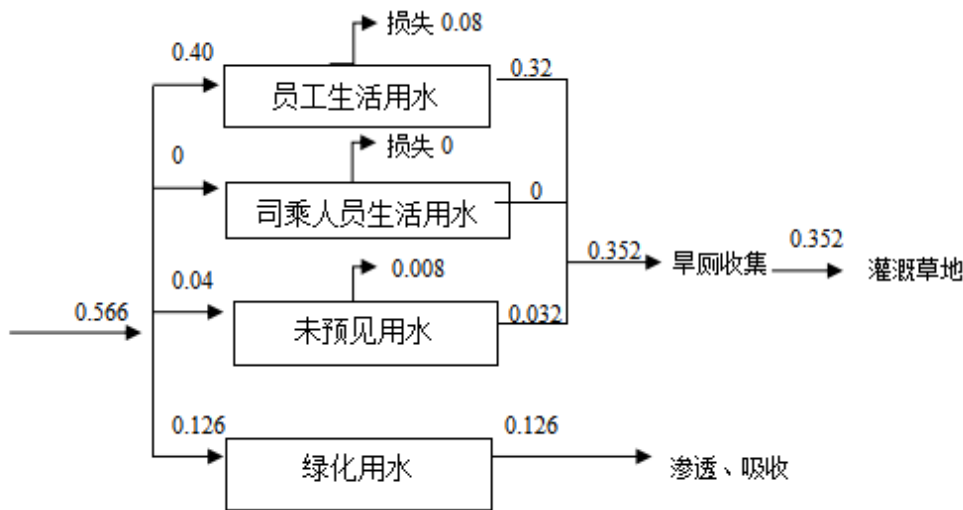
图 2-1 本项目水平衡图 单位：t/d
