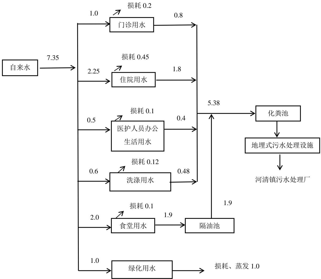
图 1-1 项目水平衡图 (m³/d)
