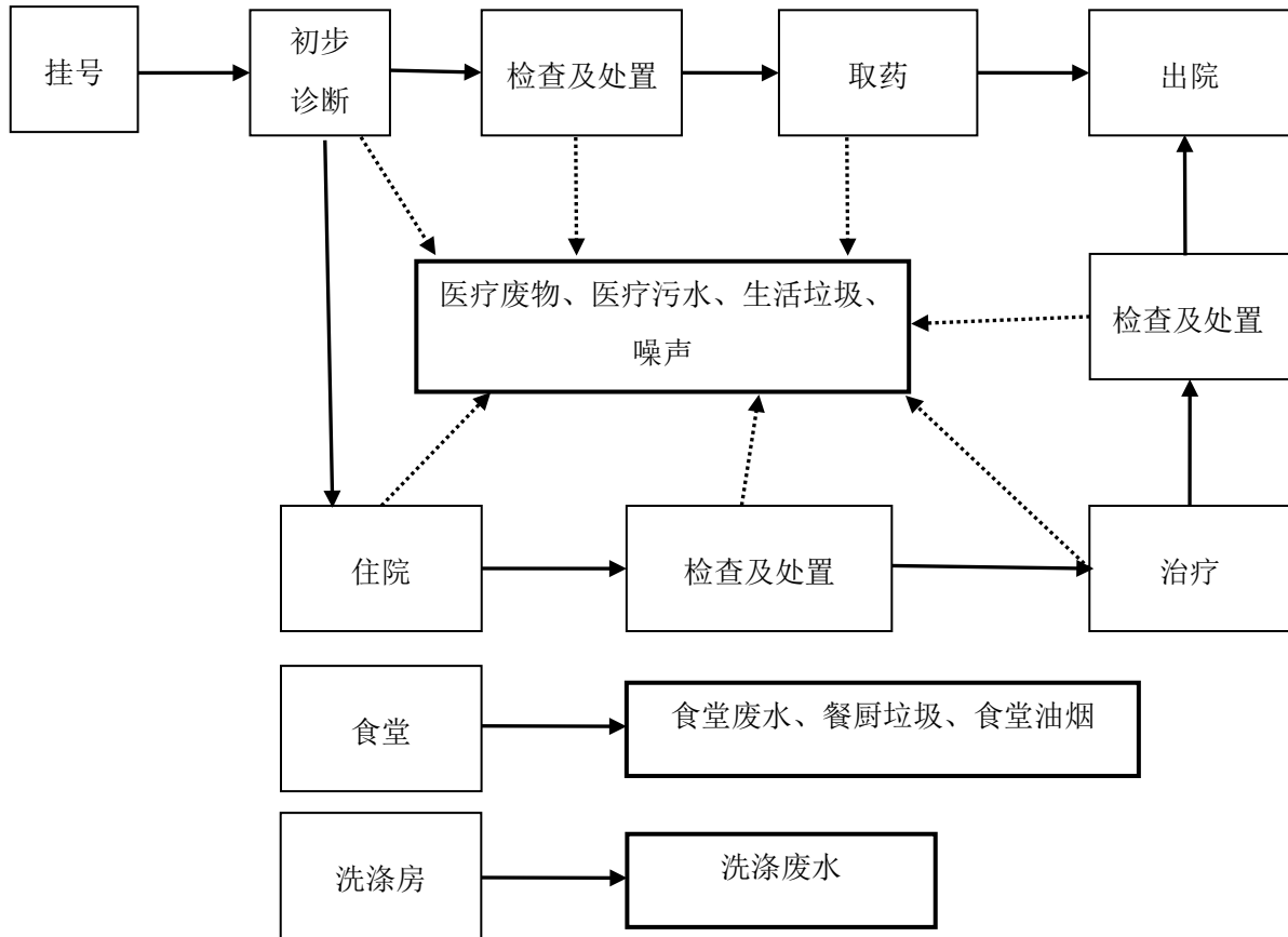
图 2-2 运行期流程及产污节点图
